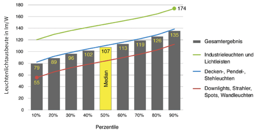
1 Häufigkeitsverteilung der Leuchteneffizienz (10000 Leuchten im Jahr 2022)
