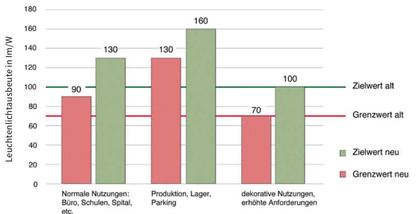
2 Anforderungen an die Leuchteneffizienz für SIA-Grenz- und Zielwerte.
