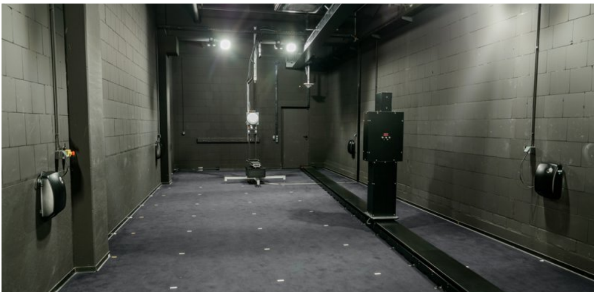
Abbildung 37: im Messraum wird mit einem normierten Dummy der Erfassungsbereich eines Sensors vermessen.
