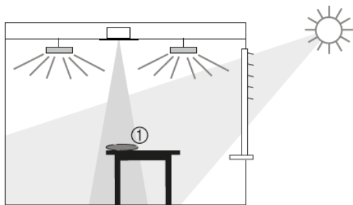
Abbildung 7: Die Lichtmessung erfolgt im Sensor an der Decke. Durch die Reflexionen des Tages- und Kunstlichtes sind die Lichtverhältnisse am Sensor nicht die gleichen wie auf dem Boden oder einem Tisch.
