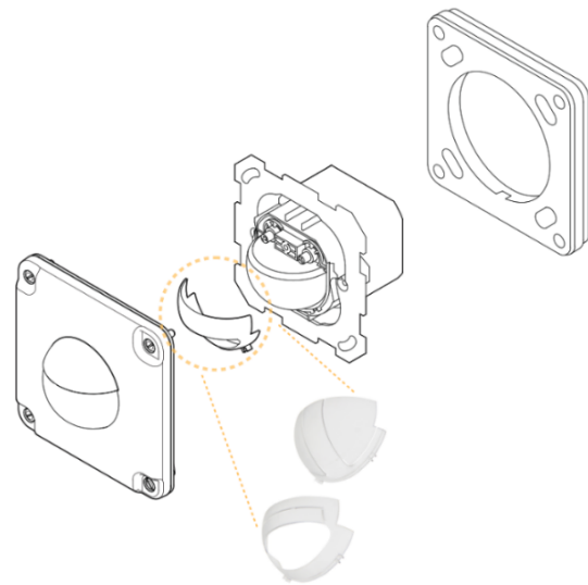
Abbildung 28: Abdeckclips ermöglichen die Begrenzung des Erfassungsbereichs eines PIR-Sensors.
