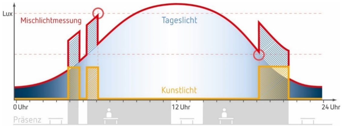
Abbildung 9: Mischlichtmessung: Der Präsenzmelder misst die Summe aus Kunst- und Tageslicht und schaltet entsprechend das Kunstlicht "EIN" bzw. "AUS".
