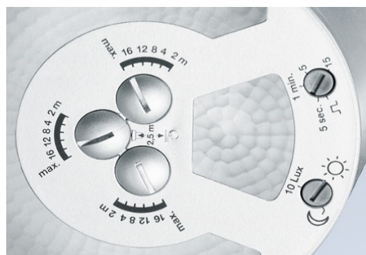
Abbildung 25: Reichweitereinstellung der Pyrosensoren durch Potentiometer
