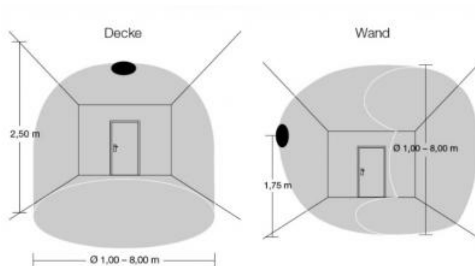
Abbildung 26: Beispieldarstellung der Erfassungsbereiche der HF-Technologie bei Wand- und Deckenmontage
