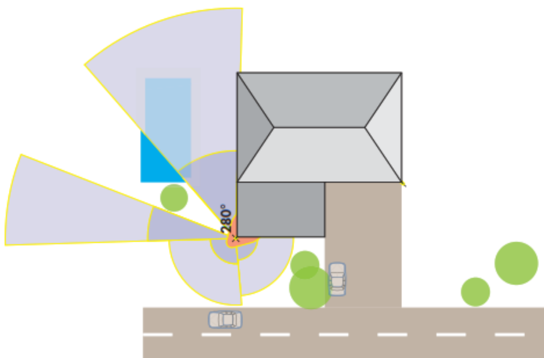
Abbildung 29: Bewegungsmelder wie hier der B.E.G. Luxomat RC-plus 280 verfügen über mehrere Sektoren, welche einzeln in der Reichweite justiert werden können. Zudem können mit Hilfe von Abdeckclips Störquellen wie Bäume oder Büsche ausgeblendet werden.
