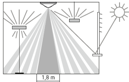
Abbildung 8: Der Raum-Korrekturfaktor bildet das Verhältnis des Lichtes an der Decke zum Licht auf der Arbeitsfläche ab.
