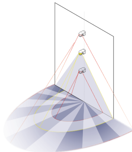
Abbildung 13: Mit zunehmender Höhe wird der Erfassungsbereich grösser und die Empfindlichkeit geringer
