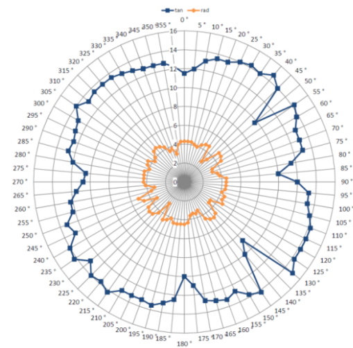
Abbildung 38: Das Polardiagramm bildet die Messergebnisse der tangentialen (blau) und radialen (orange) Erfassung eines Deckenmelders ab
