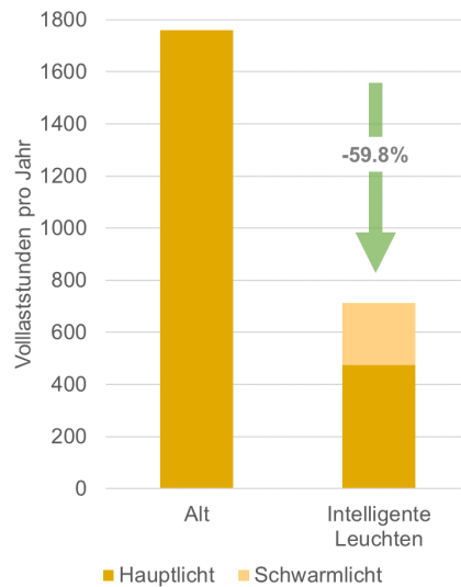
Abbildung 4: Reduktion der Brenndauer durch eine moderne Lichtsteuerung
