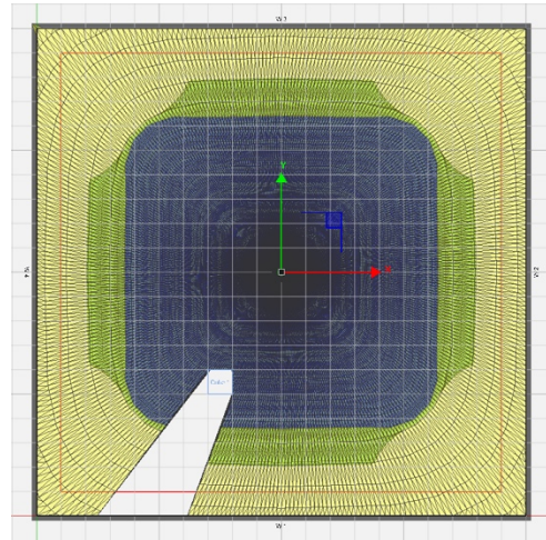
Abbildung 42: Beispiel einer Planung in RELUX mit dem IR Quattro HD von STEINEL (Aufsicht)
