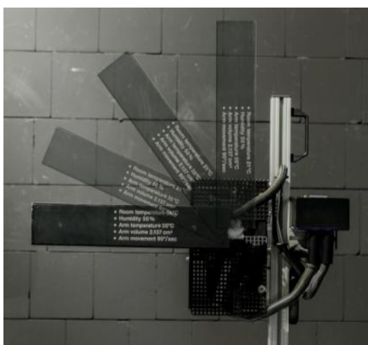
Abbildung 39: Modellarm für die Vermessung des Präsenzbereiches
