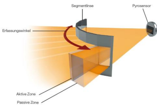
Abbildung 12: Schematische Darstellung der Erfassung eines Infrarot-Sensors
