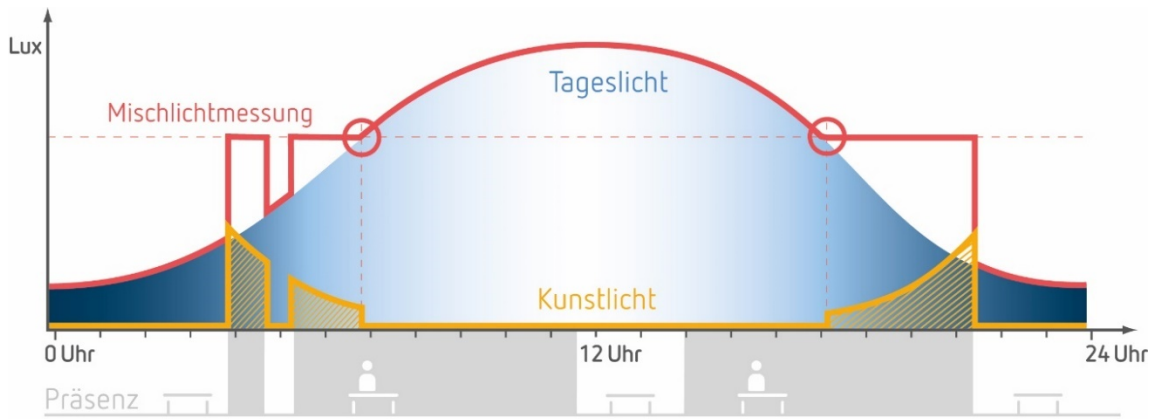
Abbildung 10: Konstantlichtregelung: Es wird nur so viel Kunstlicht wie benötigt zugeschaltet und stufenlos angepasst
