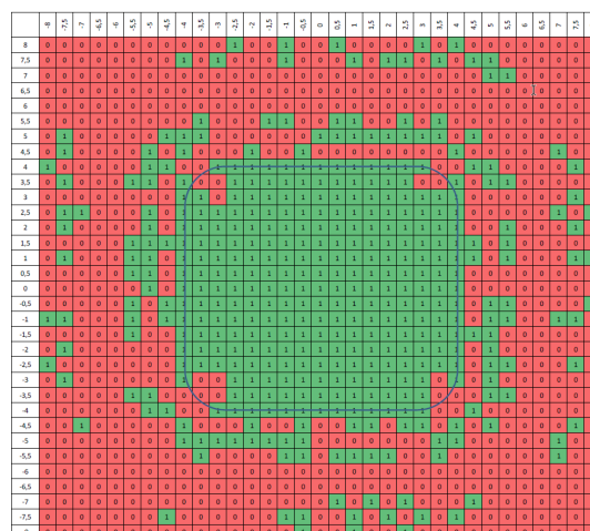
Abbildung 40: Auswertung in Rasterdarstellung einer Präsenzmessung eines Deckenmelders. Die grünen Flächen stellen die Erfassung von Präsenz dar, bei den roten Flächen gab es keine Präsenzerkennung.
