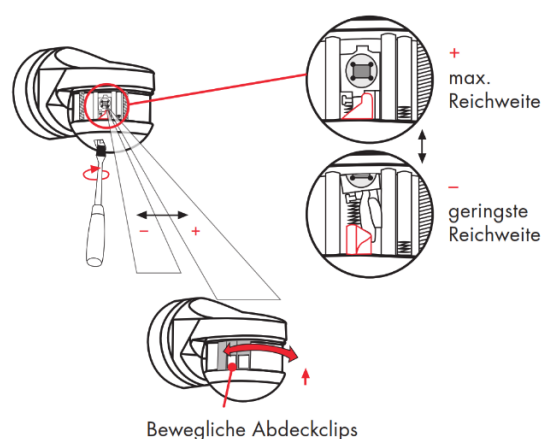
Abbildung 15: Einstellung des Erfassungsbereiches durch Drehschrauben und Abdeckclips.
