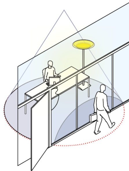
Abbildung 23: Der PIR Melder erfasst nicht durch Glaswände hindurch. Daher eignet dieser sich ausgesprochen gut für Büros mit Verglasungen.
