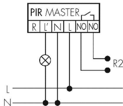
Abbildung 33: für die Ansteuerung von HLK steht ein potentialfreies Relais zur Verfügung
