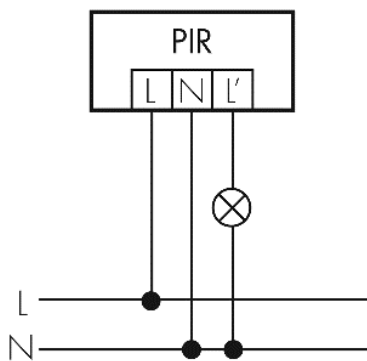
Abbildung 32: Schaltbild eines Bewegungsmelders mit einem Relaisausgang
